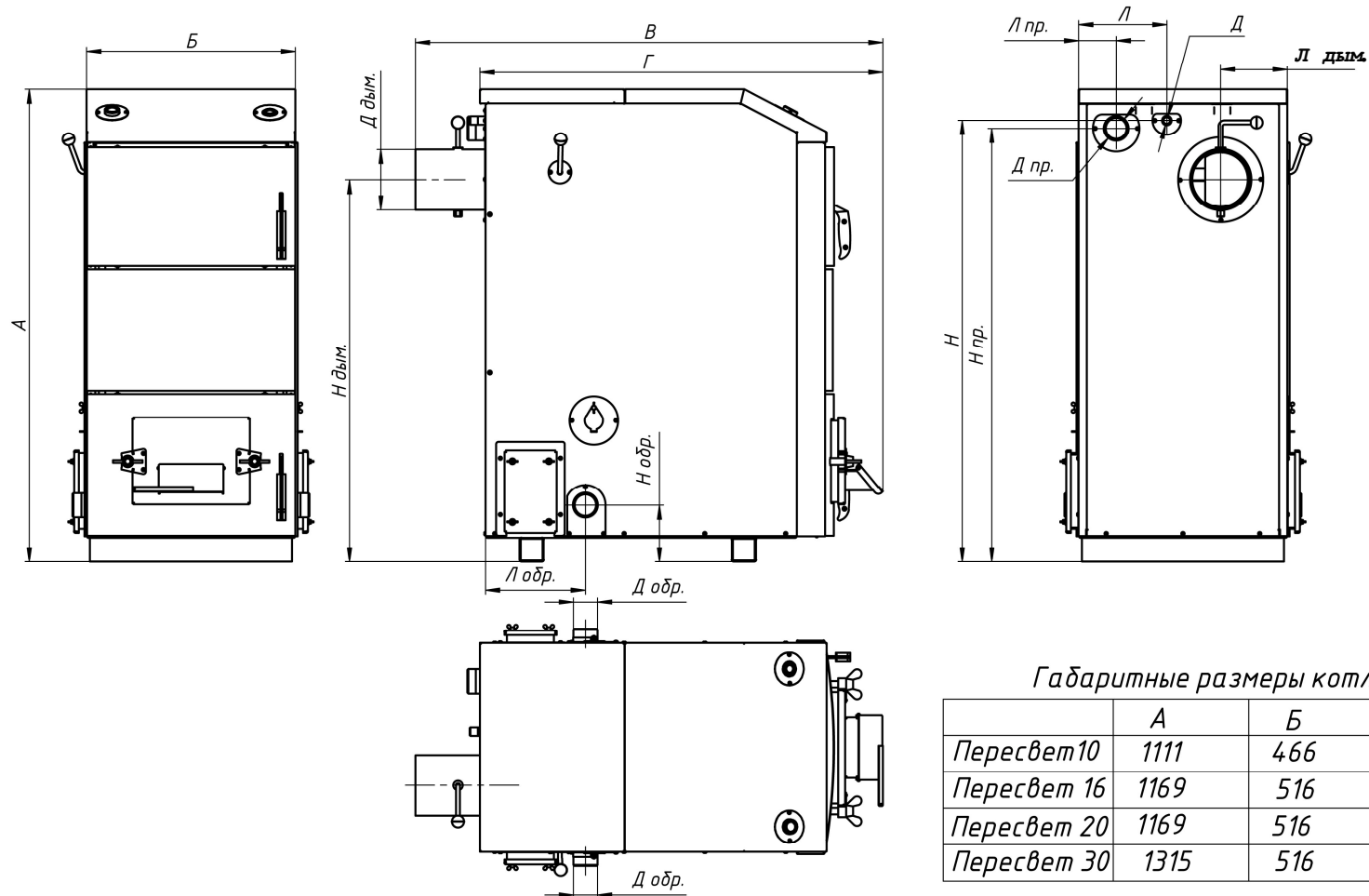
Присоединительные размеры котлов Пересвет.
